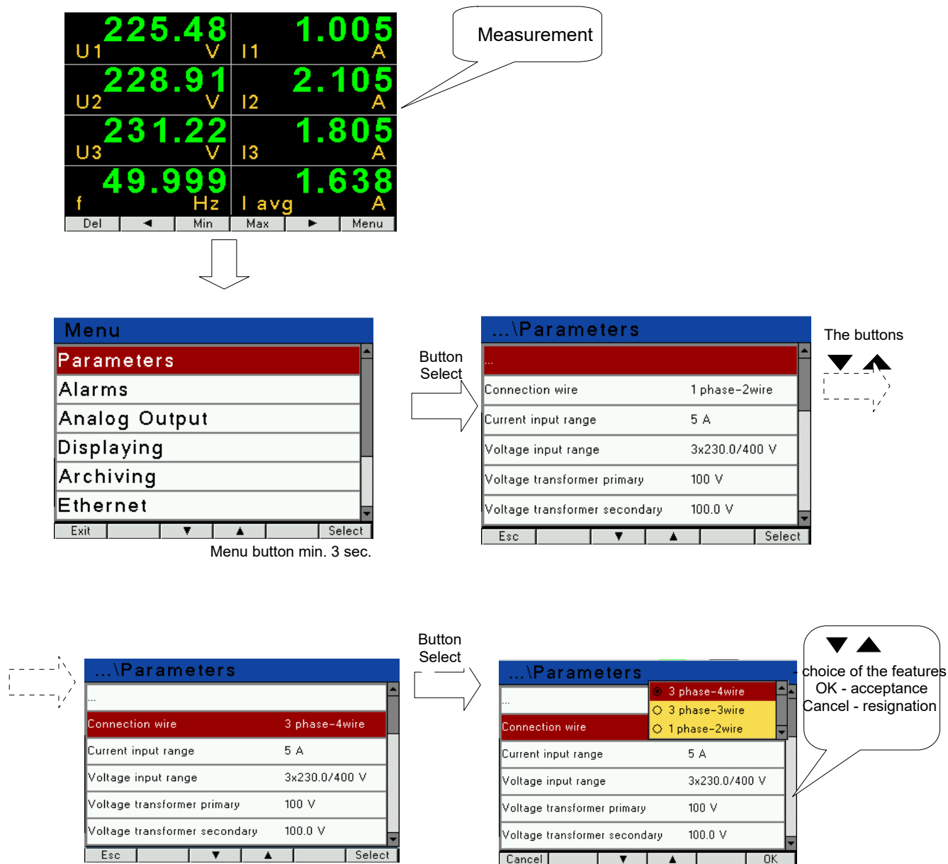
Fig. 22. Screens of Parameters mode
