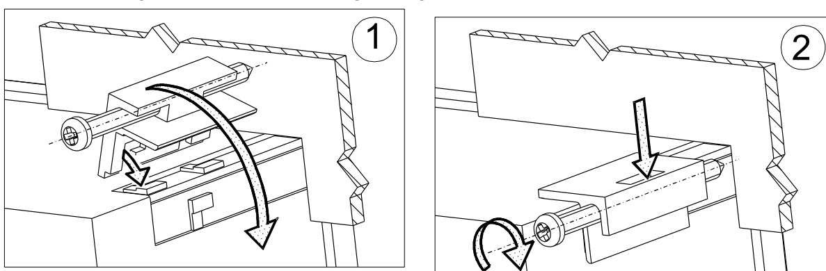
Fig. 2. Meter fitting
